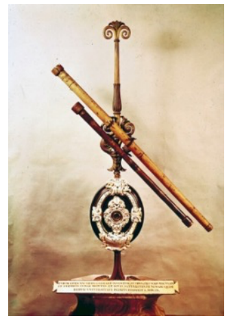
Lunette astronomique
